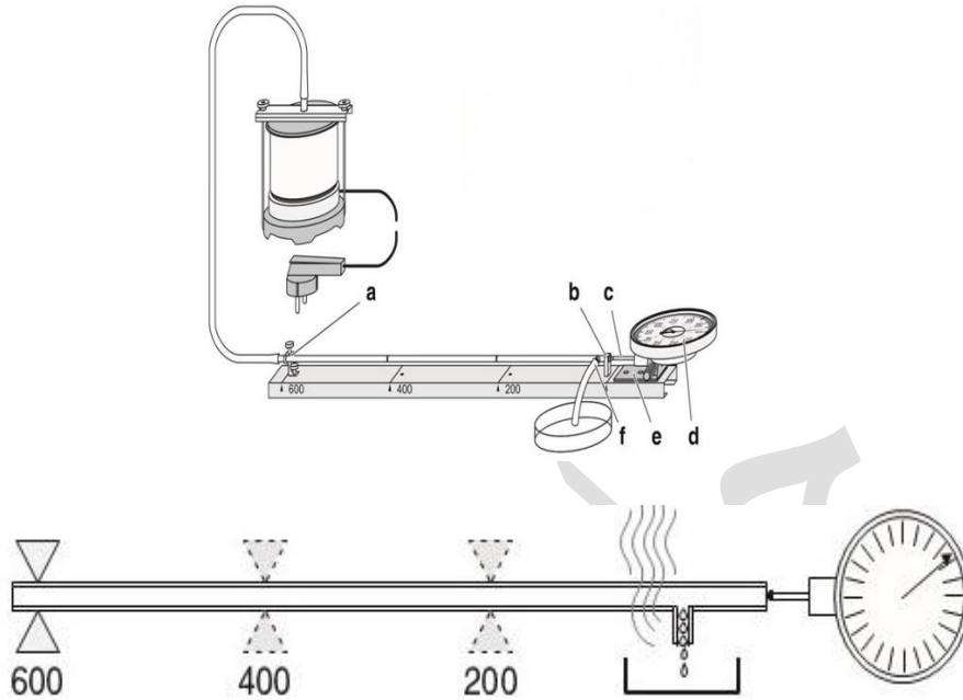
الشكل (1): رسم تخطيطي للأدوات المستخدمة في تجربة لقياس التمدد الطولي لأنبوب النحاس، كتابع لطول الأنبوب.
